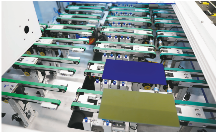
异质结电池片生产中。
