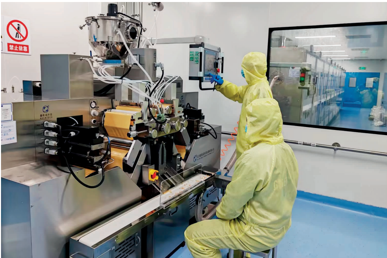
在四川国为制药有限公司制剂车间,生产工人使用全自动软胶囊机进行压丸工序的操作。
